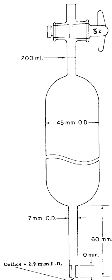
FIG. 1 Foam Pipet
